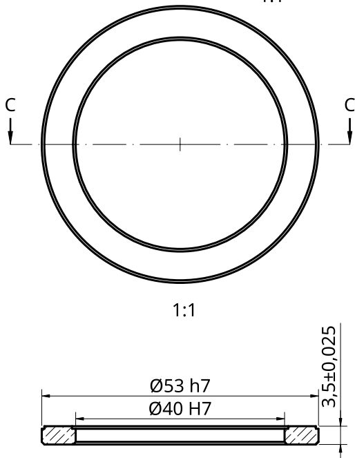
C - C 1:1
